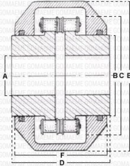
DIMENSIONES NORMA INGLESA-BS- (Tipo Renold)
