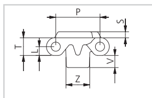
uni S-MPB C TAB con recubrimiento de caucho Dimensiones
