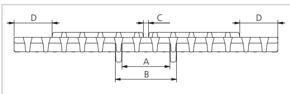
uni S-MPB C TAB con recubrimiento de caucho
